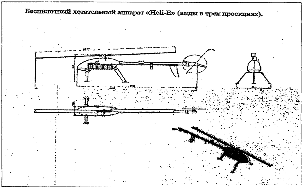
Рисунок 1. Изображение БЛА «Heli-E» ООО «Альфа Орион»
